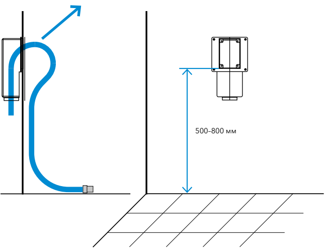
^ Интегрированный шланг Блицард Люфттехник Н-2 вытягивается вверх. Прокладка трубопровода в стяжке пола
