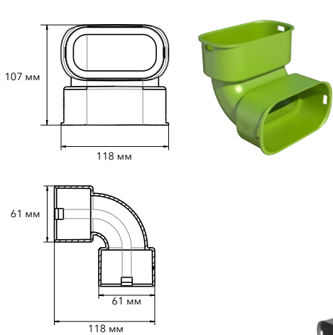
Отвод 90° вертикальный 50×102 мм ПП 630923
