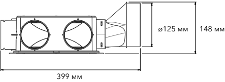
^ С соединительным комплектом Blizzard Ø 125 мм
