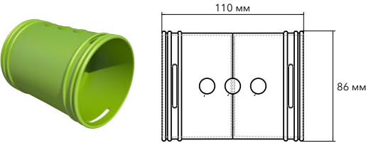
Муфта Ø 75/63 мм ПП 630973
