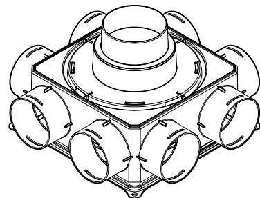
^ Коллектор Blizzard 208 8x со ступенчатым адаптером Ø 100-125 мм
