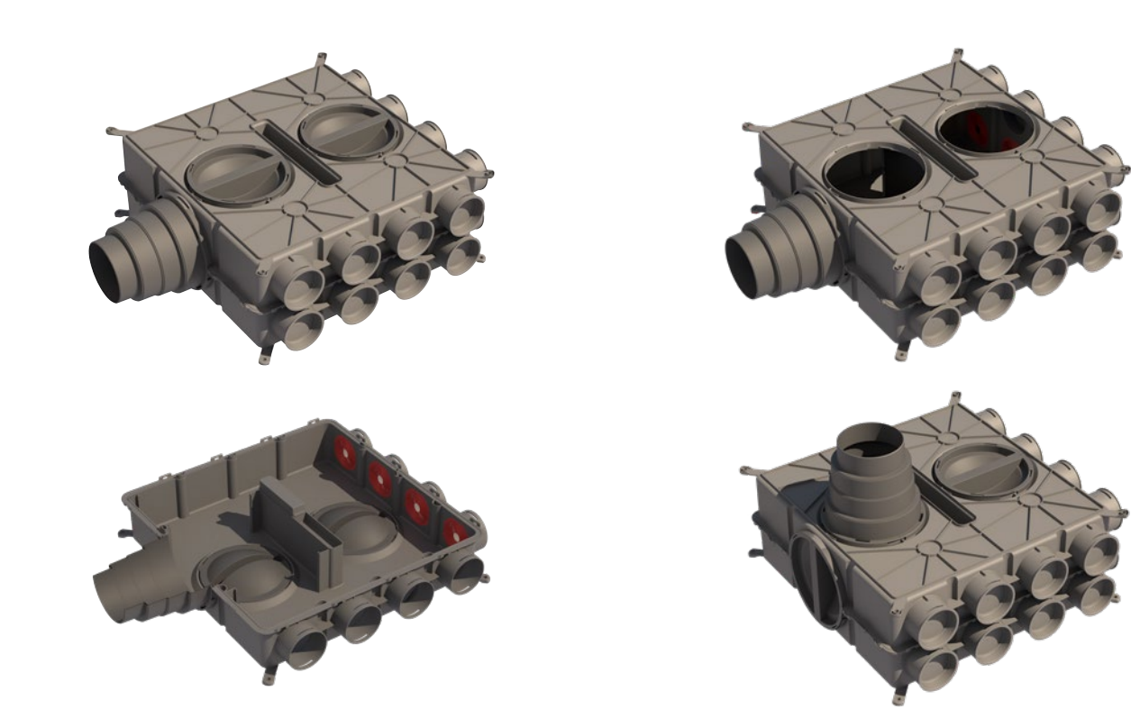
Коллектор Blizzard 816 16x Ø 75/63 мм ПП 630998
