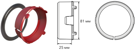
Кольцо уплотнителя Ø 75/63 мм рез. 630974SET10
