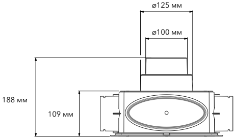
^ Со ступенчатым адаптером Blizzard Ø 100-125 мм
