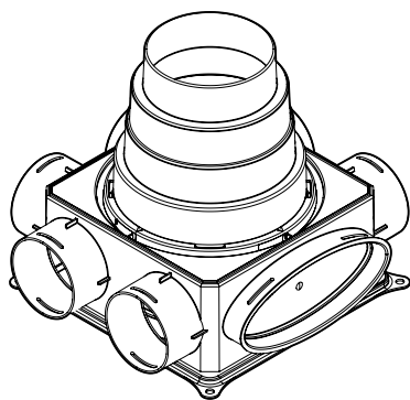
^ Коллектор Blizzard 206 6x со ступенчатым адаптером Ø 125-180 мм
