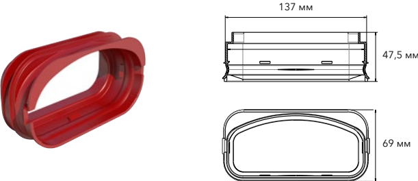
Уплотнитель 60×132 мм ПП 630932
