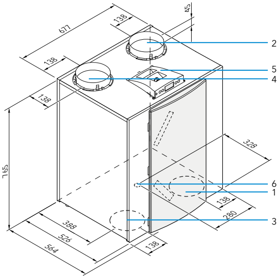
∧ RE левосторонний 2/2
