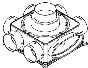
^ Коллектор Blizzard 206 6x со ступенчатым адаптером Ø 100-125 мм
