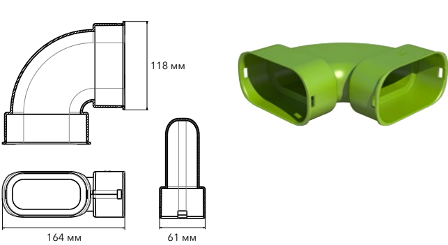
Отвод 90° горизонтальный 50×102 мм ПП 630924
