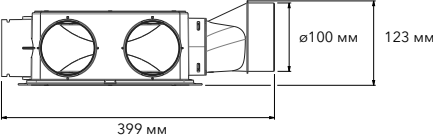
^ С соединительным комплектом Blizzard Ø 100 мм
