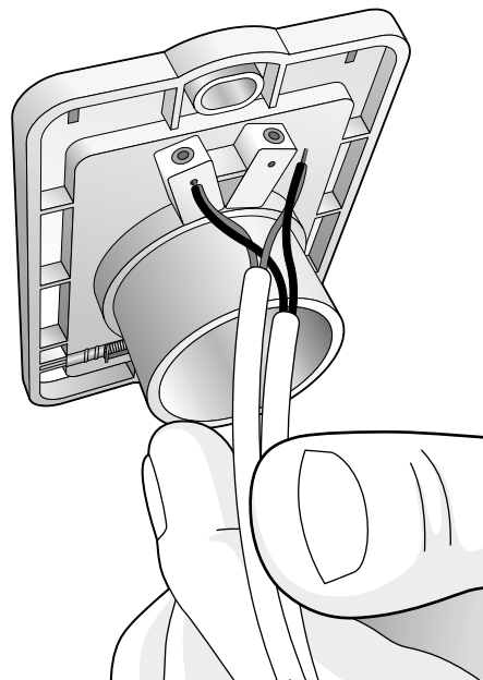
^ Подсоединение провода линии управления
