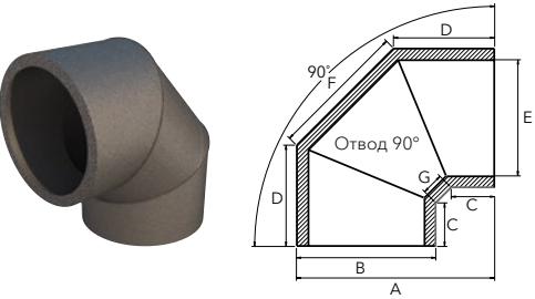
Отвод 90° Блицард
