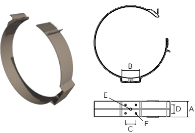
Хомут монтажный термозащитный Blizzard
