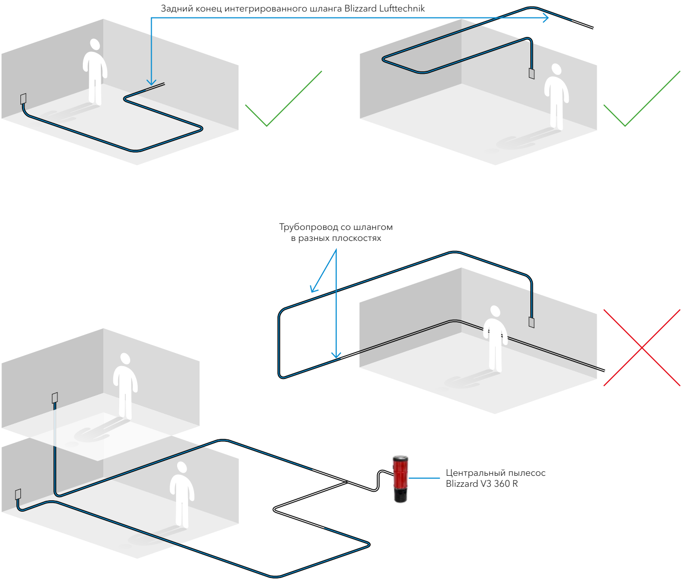
^ Прокладка трубопровода интегрированного шланга Блицард в стяжке. Шланг вытягивается вверх.
