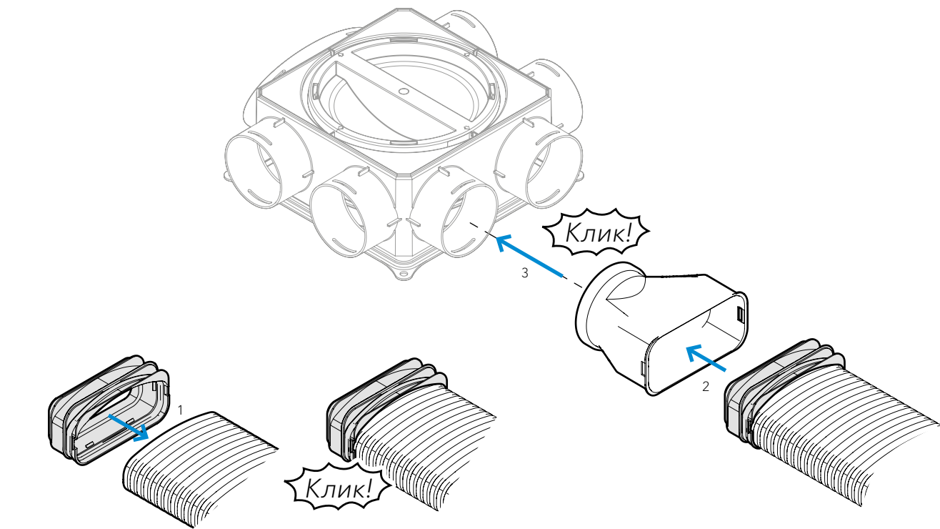
Монтаж зелёной серии Blizzard 50×102 мм и 60×132 мм
