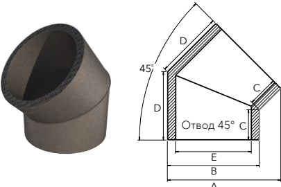
Отвод 45° Блицард
