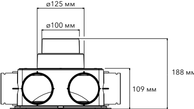
^ Со ступенчатым адаптером Blizzard Ø 100-125 мм
