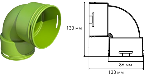
Отвод 90° Ø 75/63 мм ПП 188173
