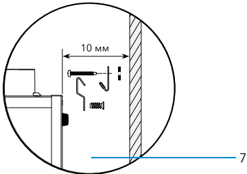
∧ Кронштейн для настенного монтажа в сборе
