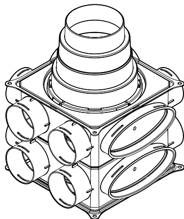
^ Вертикальное соединение коллекторов 206
