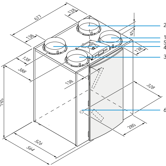
∧ RE левосторонний 4/0
