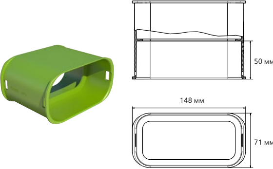
Муфта 60×132 мм ПП 630936
