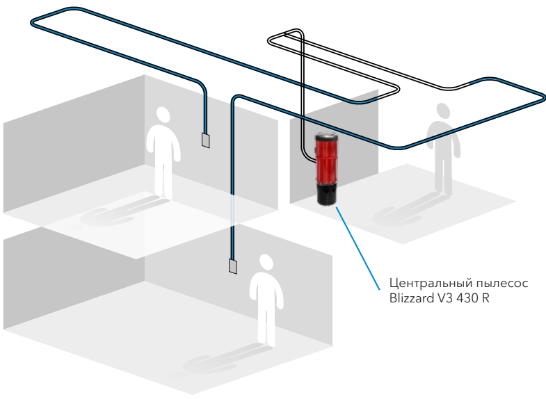
^ Прокладка трубопровода под потолком. Шланг вытягивается вниз. Требуется мощный пылесос Blizzard.
