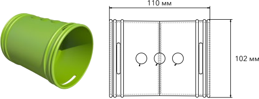
Муфта Ø 90/75 мм ПП 630983
