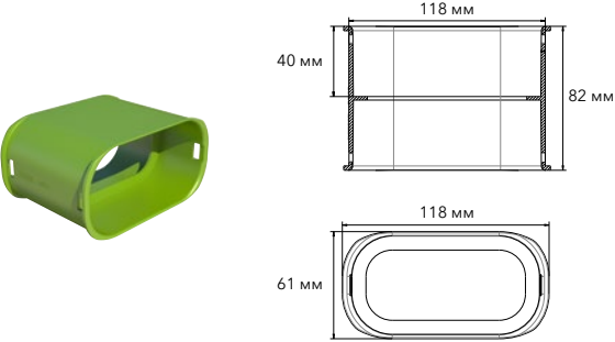
Муфта 50×102 мм ПП 630926
