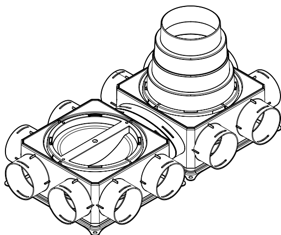
^ Горизонтальное соединение коллекторов 206
