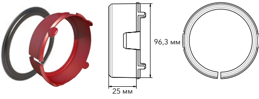
Кольцо уплотнителя Ø 90/75 мм рез. 630982SET10
