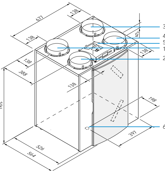
∧ RE правосторонний 4/0
