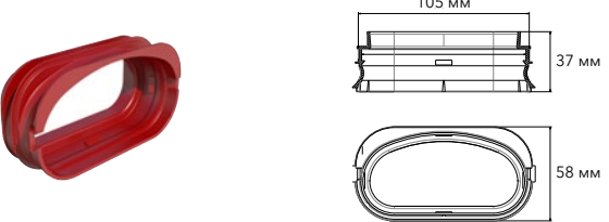
Уплотнитель 50×102 мм ПП 630922
