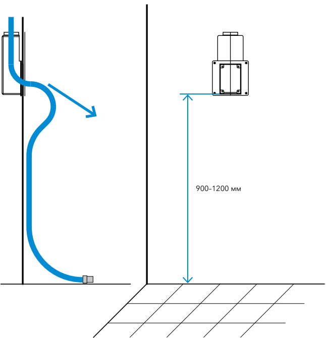
^ Интегрированный шланг Блицард Люфттехник Н-2 вытягивается вниз. Прокладка трубопровода под потолком.
