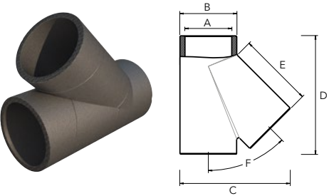
Тройник 45° Y термозащитный Blizzard
