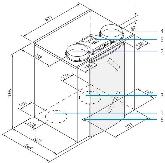
∧ RE правосторонний 2/2
